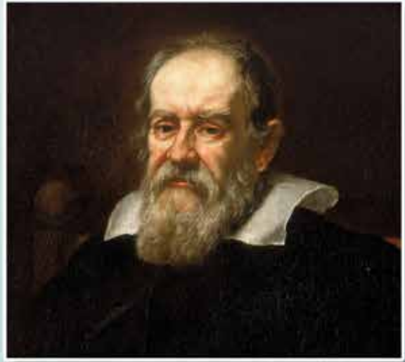
Qalileo Qaliley (1564-1642)
