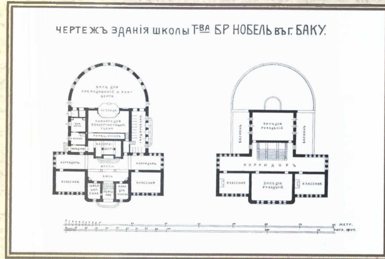
Bakıda "Nobel Qardaşları" şirkətinə məxsus məktəbin çertyoju
