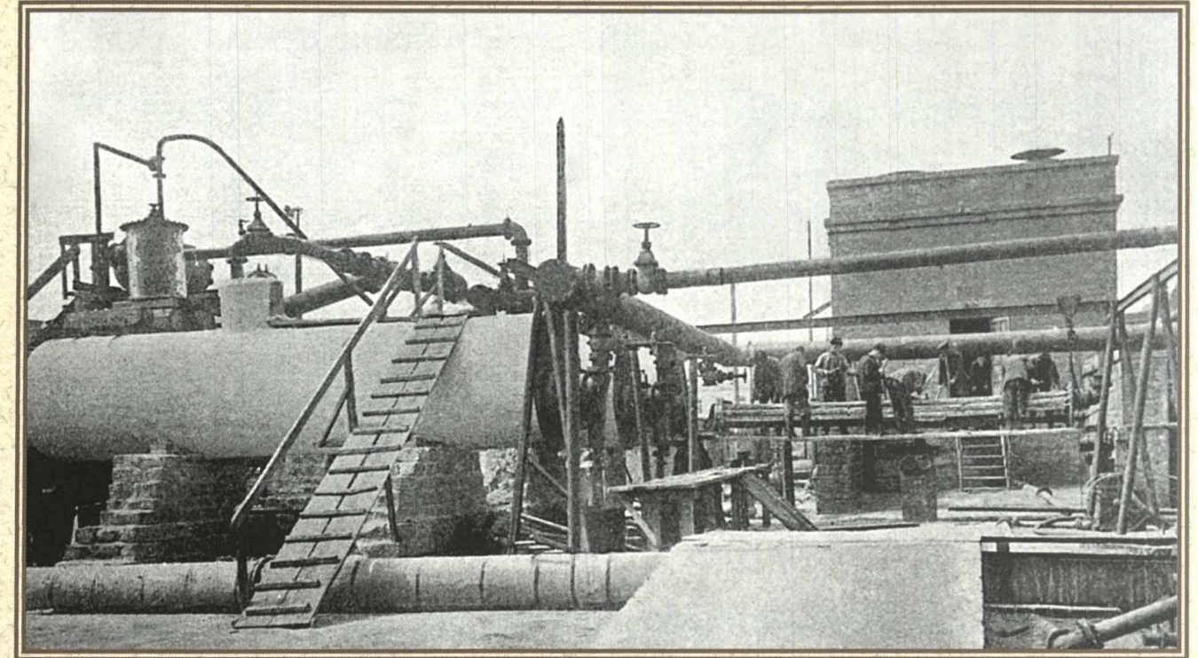
"Nobel Qardaşları" şirkətinin yağ zavodunda su təmizləyici qurğunun ümumi görünüşü
