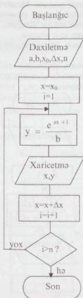
Şəkil 4.6. Dövrlər sayı verilən monoton dəyişənli hesablama prosesinin blok-sxemi
