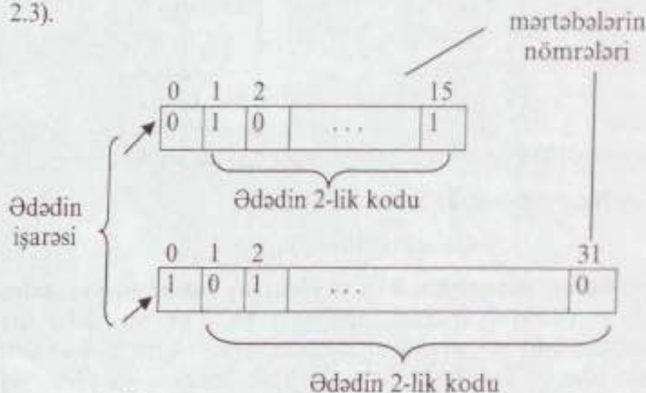
Şəkil 2.3. Tam və sabit nöqtəli ədədlərin kompüterdə təsviri
