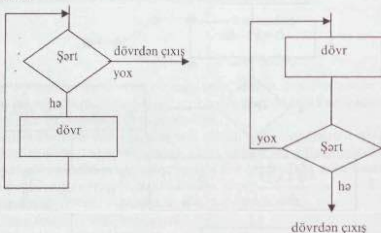
Şəkil 4.5.a. Önşərtli dövr
