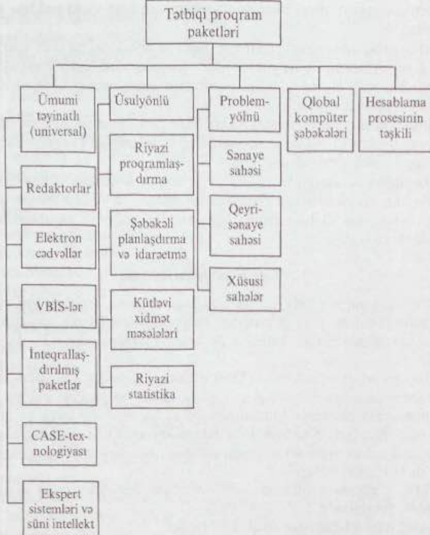
Şəkil 7.2. Tətbiqi program təminatının təsnifat sxemi
