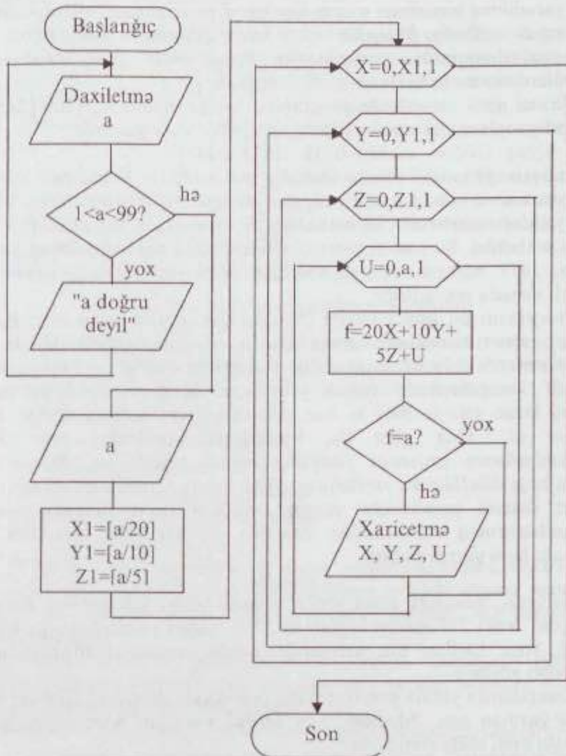
Şəkil 4.14. Məsəl 12-nin həllini təmin edən alqoritmin blok-sxemi
