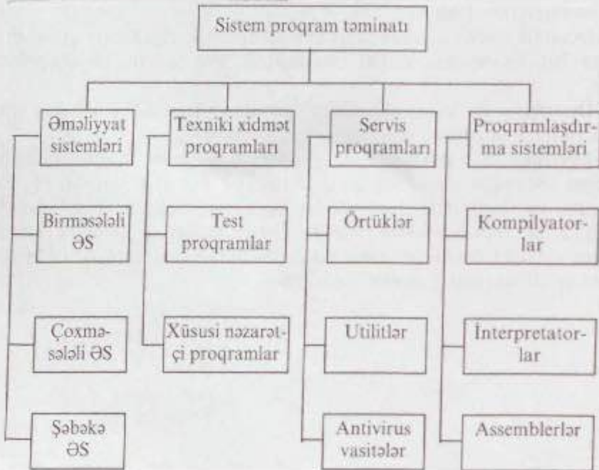
Şəkil 7.1. Sistem proqram təminatı
