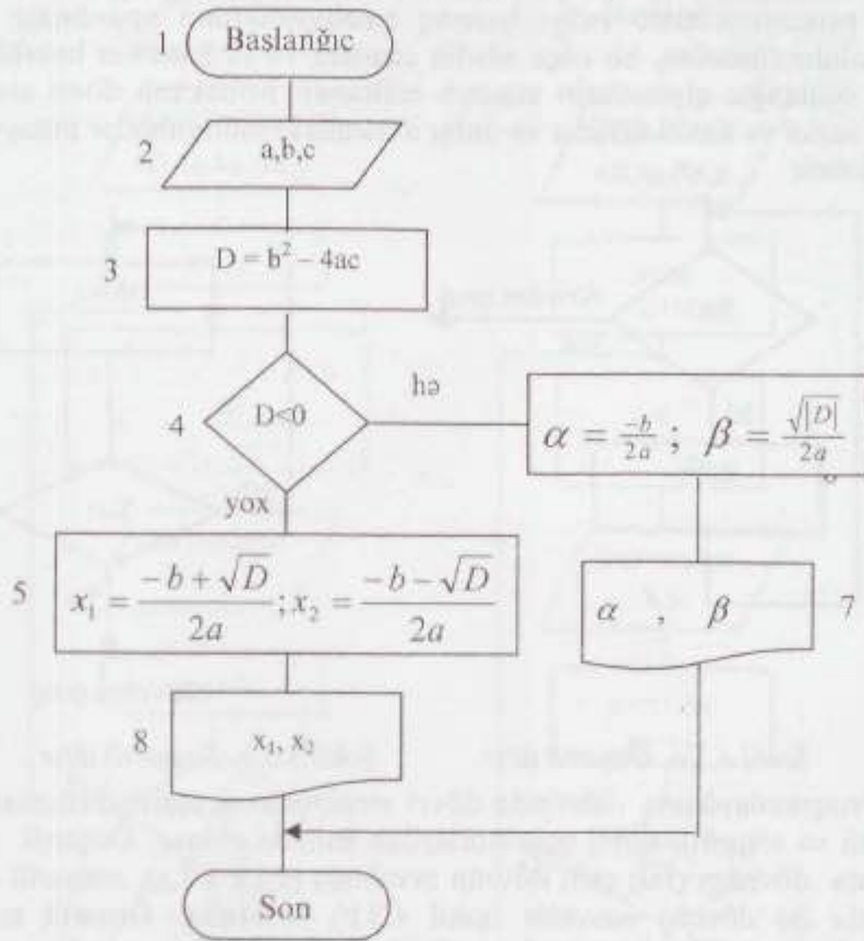
Şəkil 4.4. Kvadrat tənliyin həll alqoritmı
