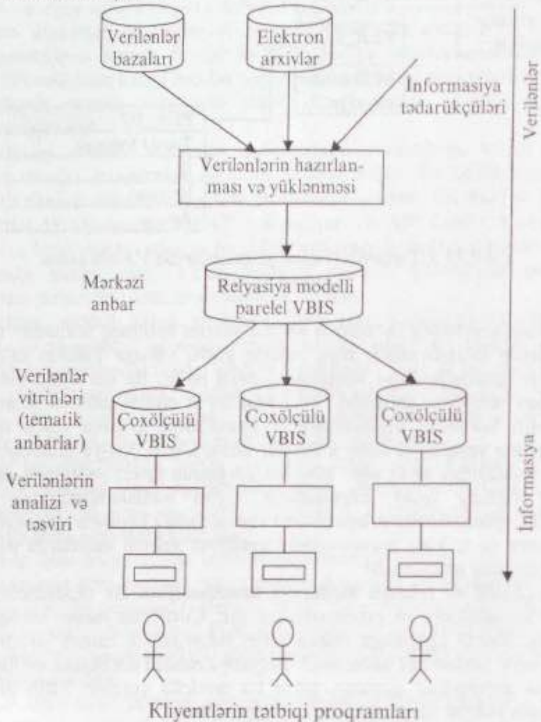
Şəkil 13.4. Verilənlər anbarlarından və verilənlər vitrinlərindən istifadə edən QQDS-in məntiqi sxemi
