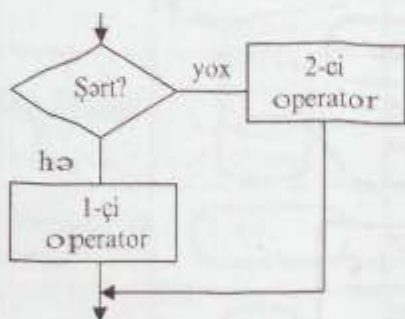
Şəkil 4.2. Tam formalı budaqlanma
