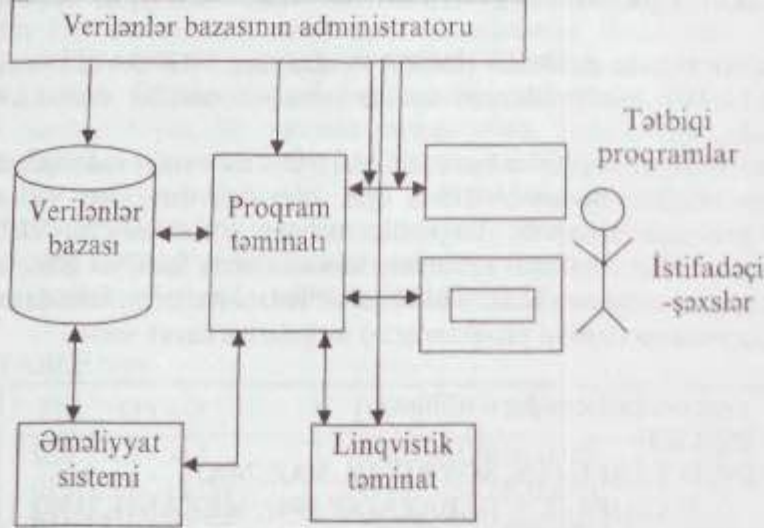
Şəkil 12.10. VBİS-in sadələşdirilmiş sxemi
