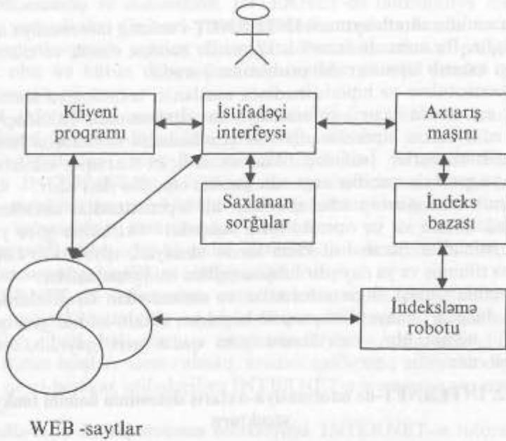
Şəkil 16.2. INTERNET-də informasiya-axtarış sisteminin tipik funksional strukturu
