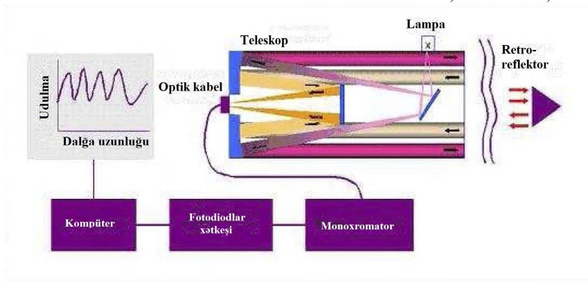
Şək. 2.7. Konsentrasiyanın DOAC-4P cihazı ilə nəzarəti
