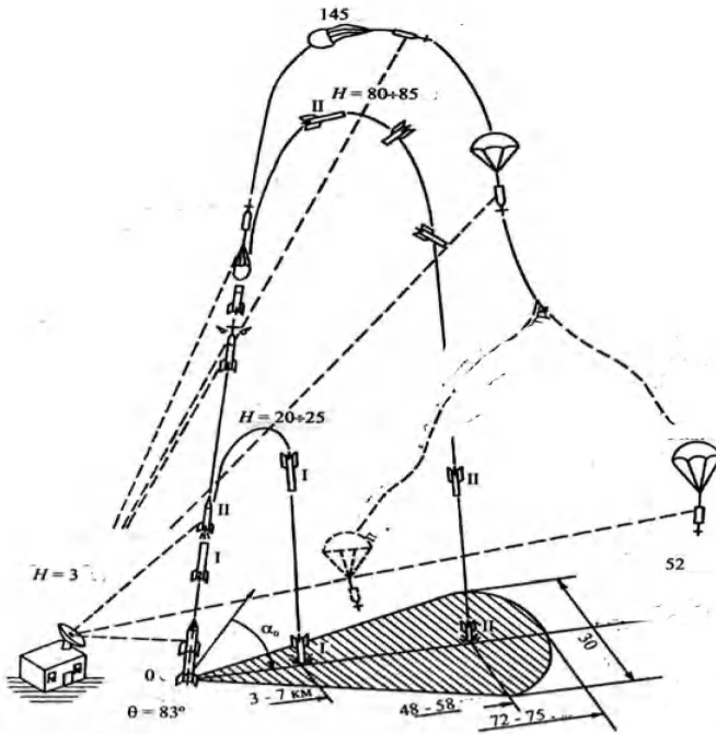
Şək.2.2. M-100B meteoroloji raketin qalxma və uçuş trayektoriyasının sxemi.
