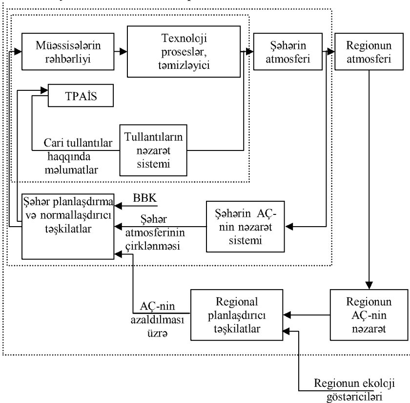
Şək.1.7. Regionun təbii mühitin vəziyyətinin tənzimləmə sisteminin strukturu.
