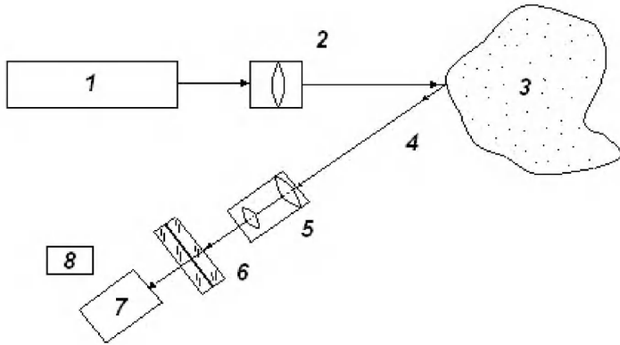
Şək.2.3 Lidarın ümumi sxemi.
