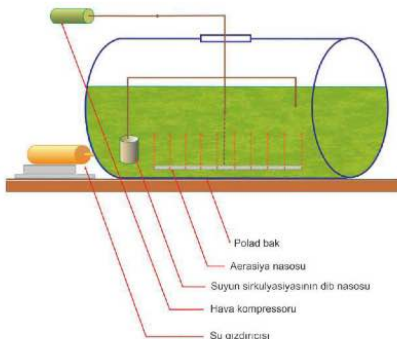
Şəkil 8.23. Biotexnologiya rekultivasiya metodunun blok sxemi
