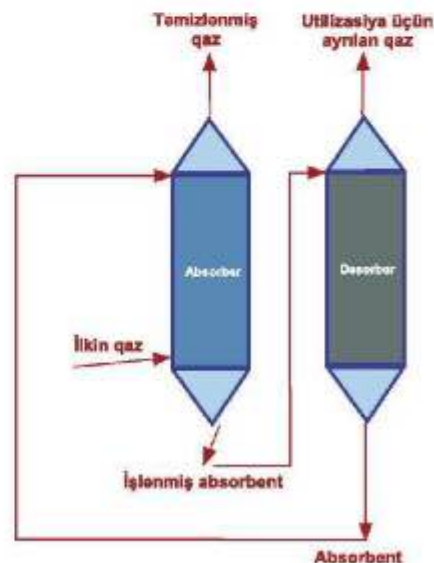
Şəkil 10.14. Absorbsiya və desorbsiya proseslərinin sxematik təsviri
