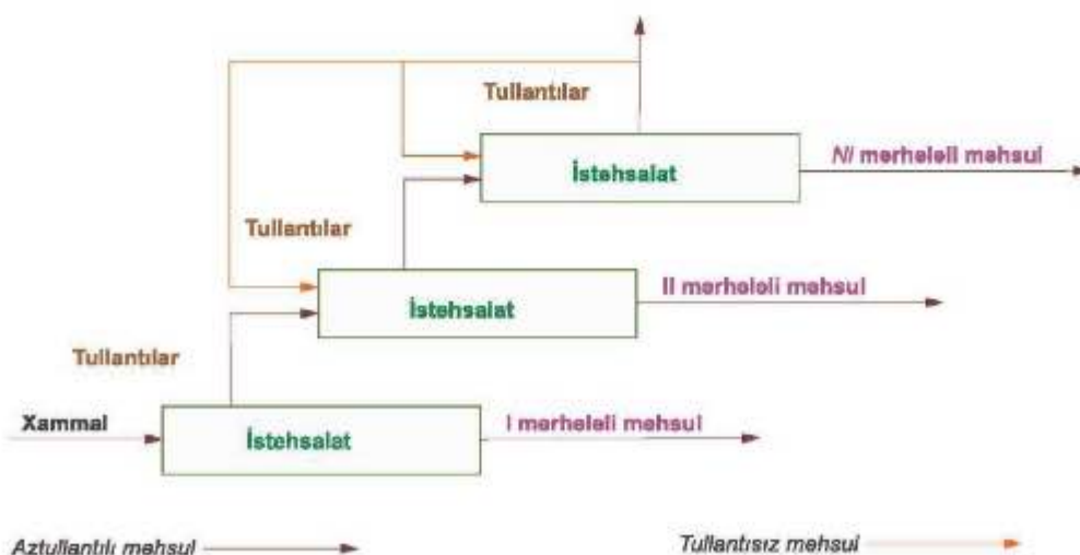
Şəkil 10.17. İstehsalın aztullantılı texnoloji sistemi
