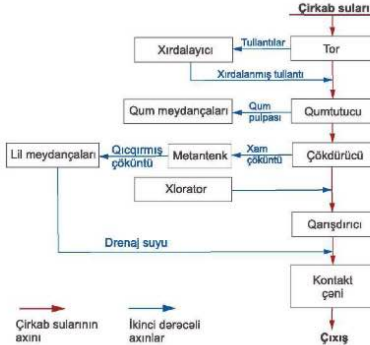
Şəkil 10.15. Çirkab suların mexaniki təmizlənməsinə əsaslanmış təmizləyici stansiyanın texnoloji sxemi
