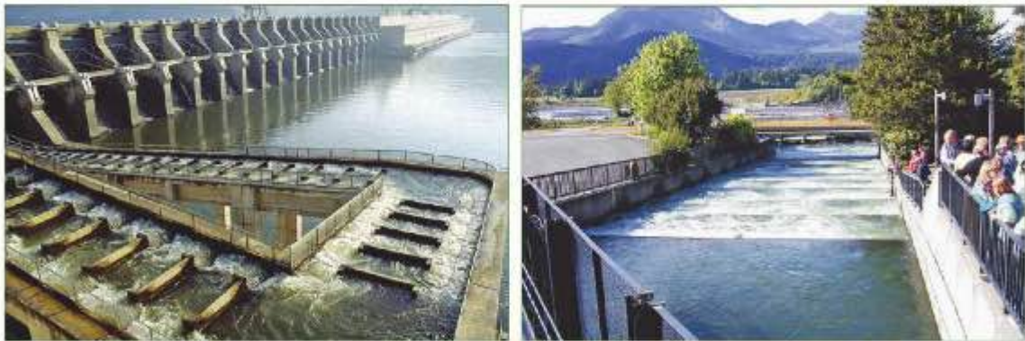
Şəkil 7.80. Kolumbiya çayında və Bonnevil bəndində quraşdırılmış balıq-keçidləri (ABŞ).
