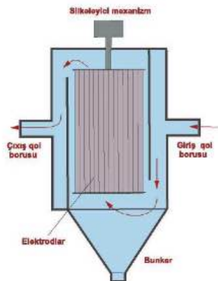
Şəkil 10.13. Lövəli elektrik filtri
