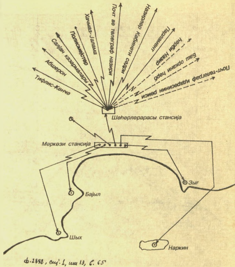
ŞƏKİL 10. Bakı İstehkamat hissəsinin rabitə şəbəkəsi
