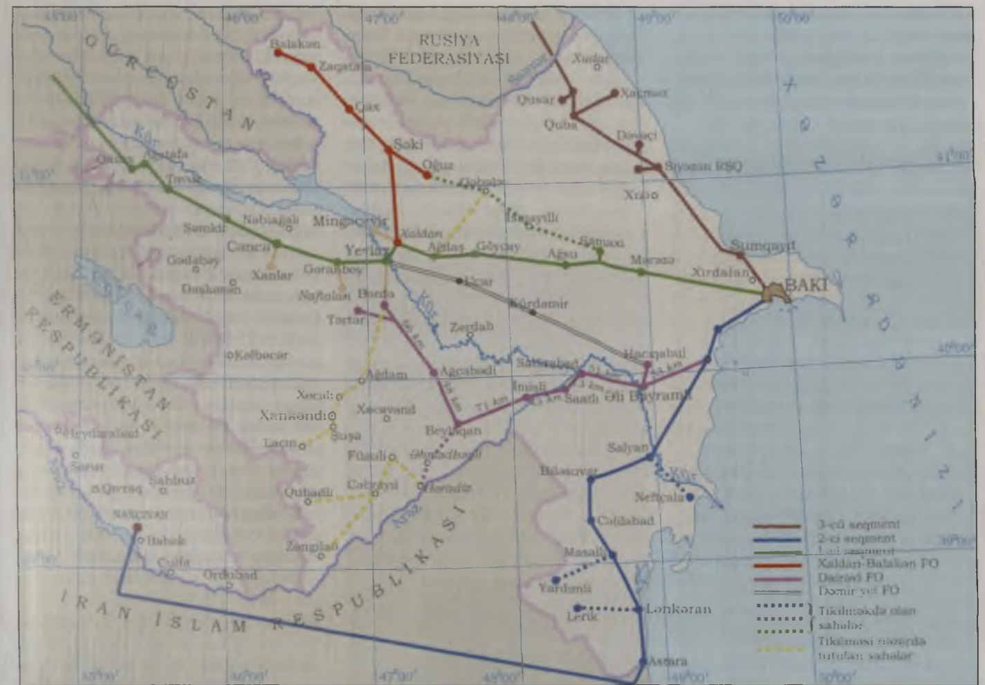
TAE fiber-optik kabel magistralının Azərbaycan seqmenti.
