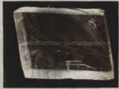
İslandiya şpatı.
