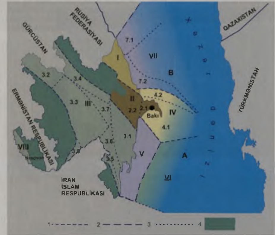
Azərbaycan Respublikasının neft-qazlıqlığa görə geoloji rayonlaşdırılma sxemi:
